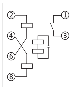
DD-11接线图
