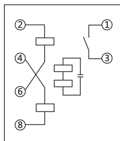
DT-1接线图
